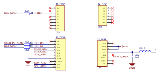
DM-TFT28-116 Display Header (optional)
